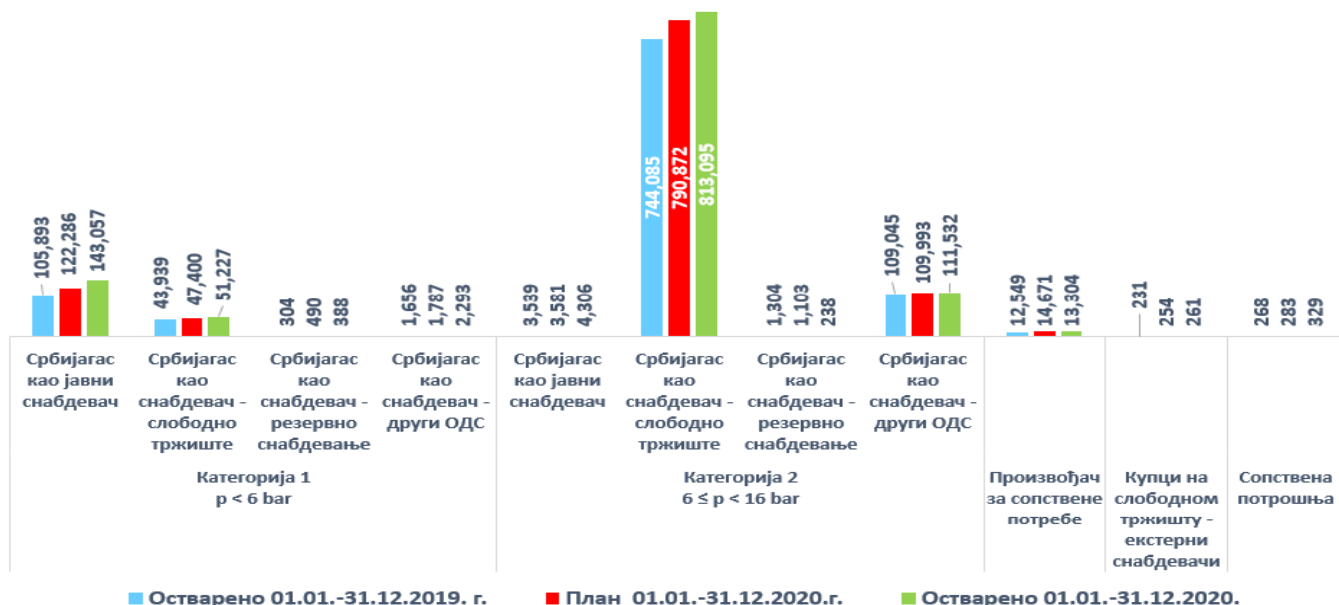
График бр. 2 , Упоредни преглед структуре снабдевања са дистрибутивног система (у 000 m³)
