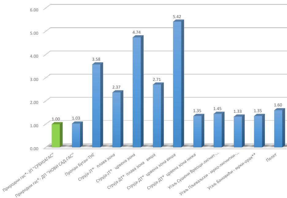
ДИЈАГРАМ СА УПОРЕЂЕНИМ ИНДЕКСИМА ЦЕНА РАЗЛИЧИТИХ ЕНЕРГЕНАТА
